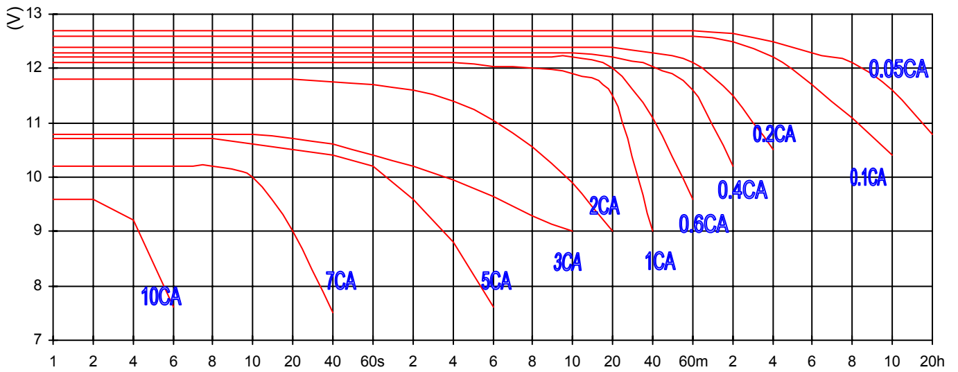
Abb.3: Entlade-Kennlinien (C=45)
